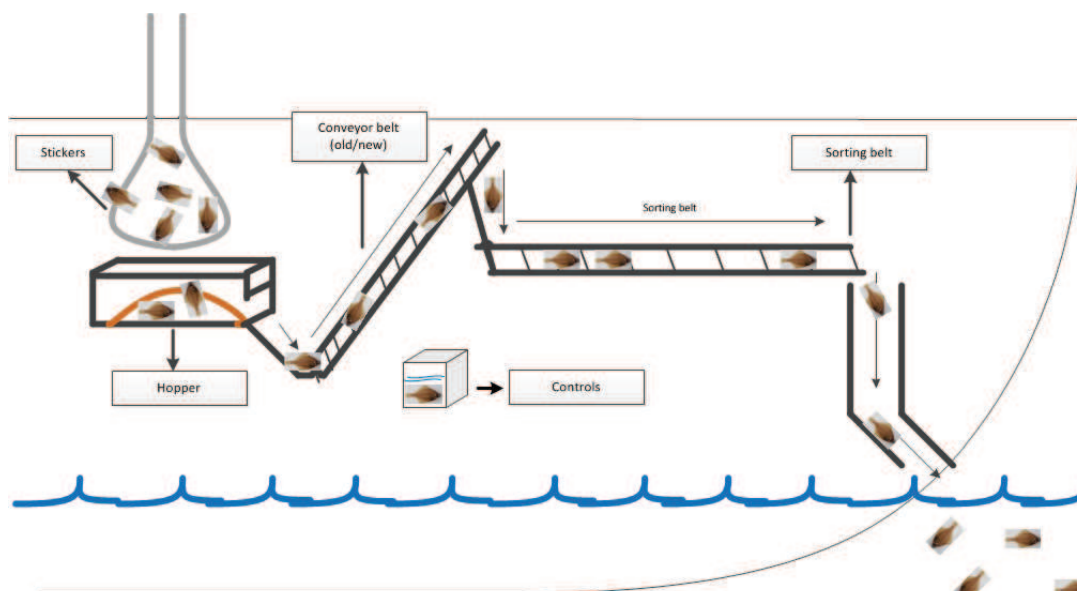
Figuur 3. Schematische tekening van de verwerkingslijn met bemonsteringslocaties voor de overlevingsproeven. Stickers : stekers door de mazen van de kuil, dit betreft alleen ondermaatse tong gedurende reis 3. Hopper - vissen uit de stortbak random verzameld direct na het storten van de vangst. Conveyor belt – dit betreft alleen vissen voor het bepalen van het effect van aanpassingen aan de stortbak op de overlevingskansen van discards (project "Verhogen"). Controls – dit zijn controlevissen afkomstig uit het lab in Yerseke, aangevoerd in een 600L tub. Sorting belt – op dit punt zijn alle vissen voor het project "Vaststellen" verzameld.
