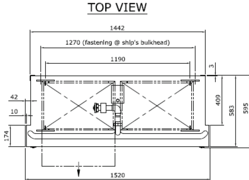
Figuur 2. Bakkensysteem bovenzijde.
