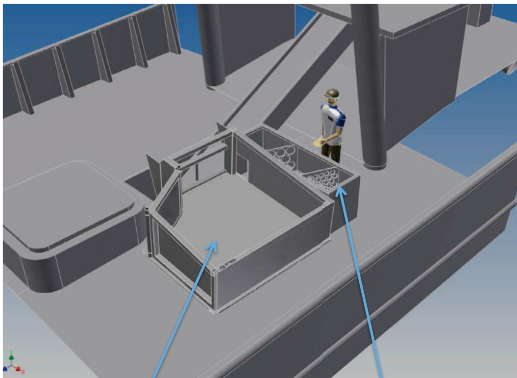
Aangepaste stortbak
